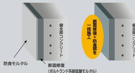
リフレドライショット（耐酸タイプ）の場合
