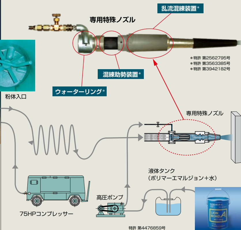
■リフレドライショットの吹付けシステム
