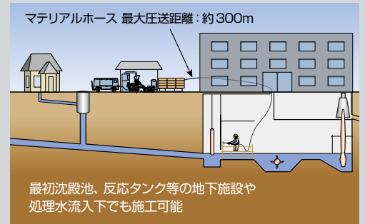
リフレドライショット（耐酸タイプ）の場合
